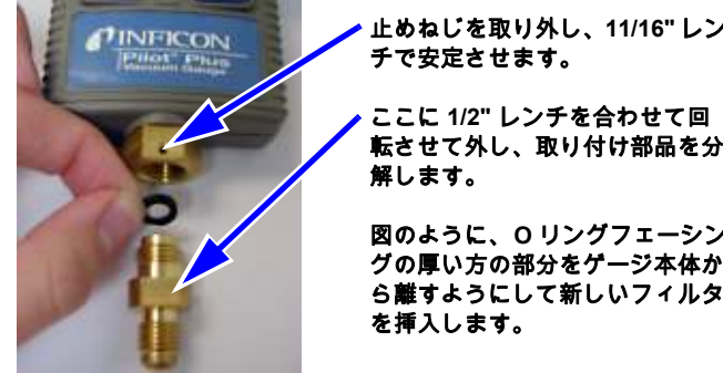
図 3. Pilot Plus 取り付け部品
